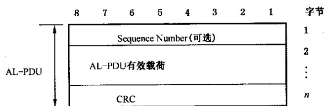
图 10 AL2-PDU 数据结构
