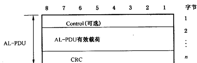
图 11 AL3 层 PDU 数据结构
