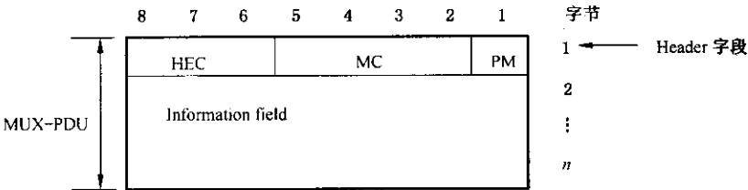
图 9 MUX-PDU 数据结构
