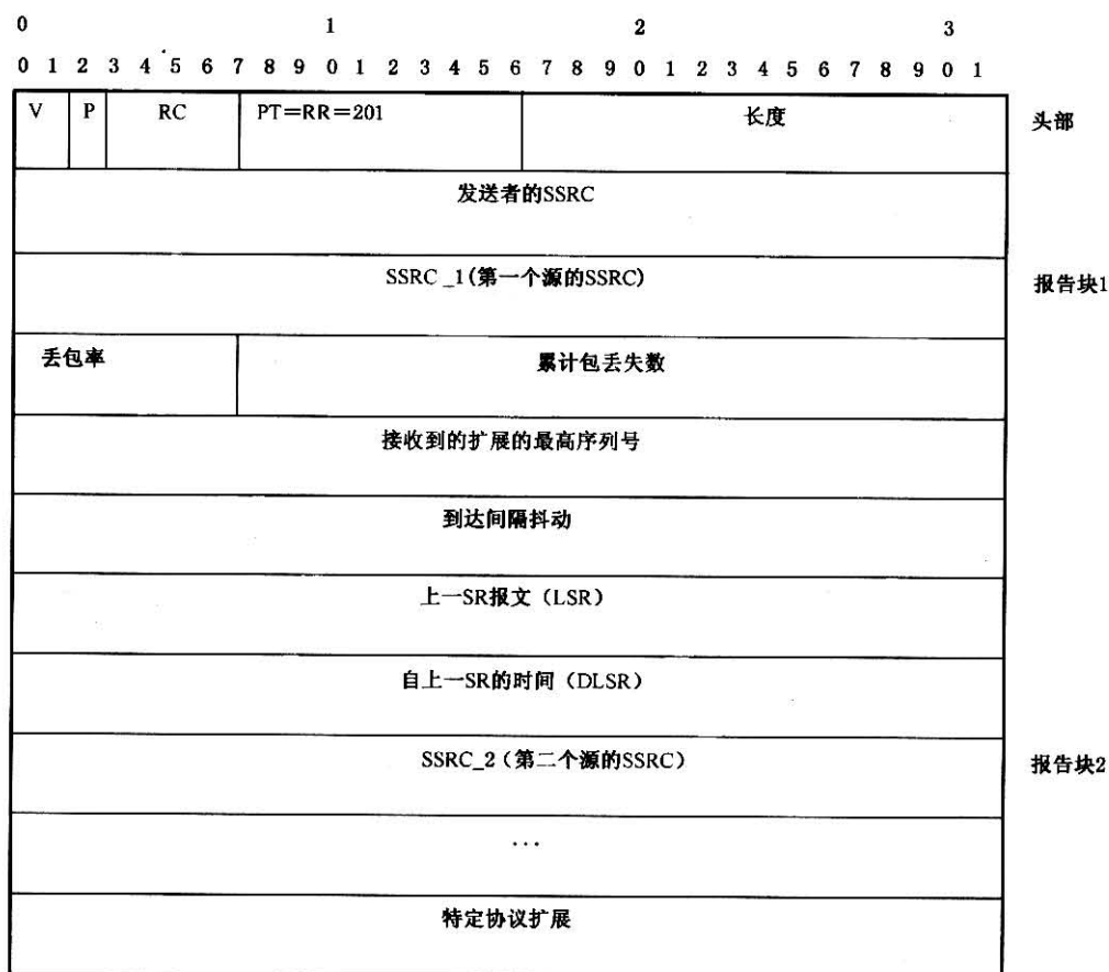
图 5 RR 报文格式
