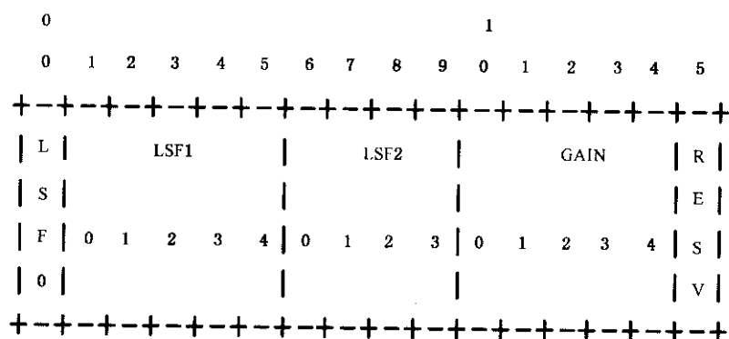
图 2 ITU-T G.729 舒适静音帧结构
