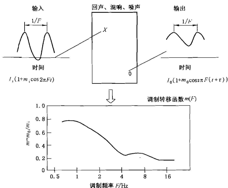
图 13 调制转移函数:输入/输出比较
