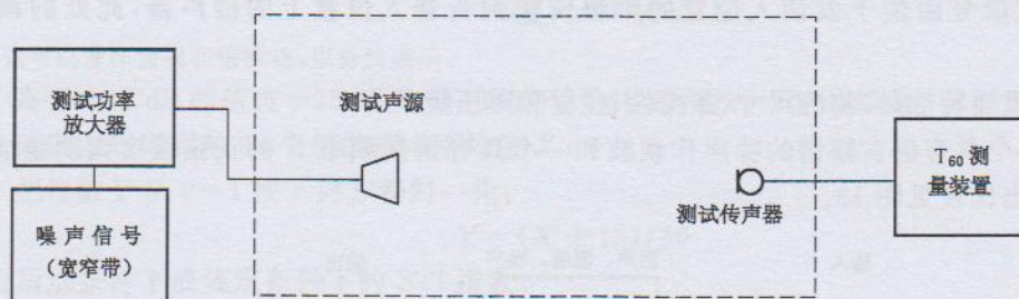
图 11 用模拟自然声源进行混响时间测量的原理框图
