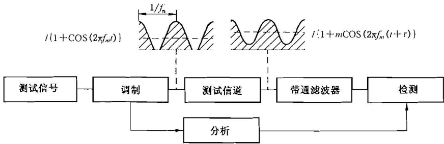
图 16 STIPA 方法测量原理框图
