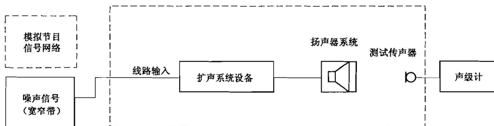
图3 电输入法测量传输频率特性原理框图
