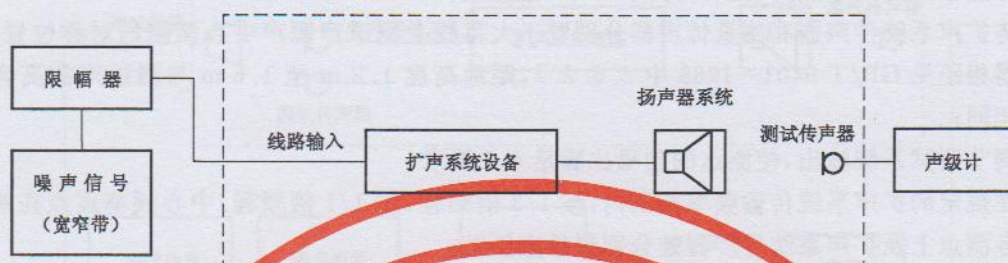
图 4 电输入法中用窄带噪声测量最大声压级原理框图
