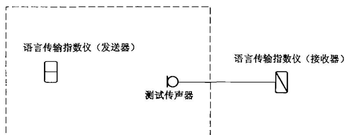
图 14 无扩声时 STI 法测量原理框图
