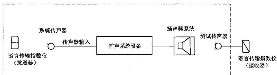
图 15 有扩声时 STI 法测量原理框图
