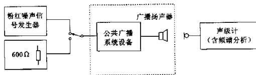
图 5.3.1 公共广播系统电声性能测量原理
