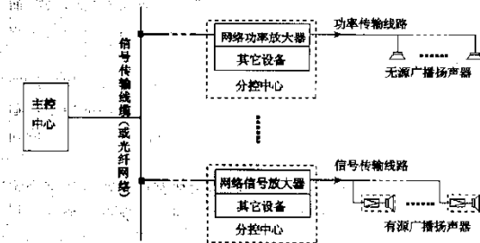
图3 有源终端和无源终端相结合的方式
